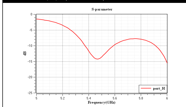
水平 (Horizontal) Return Loss
