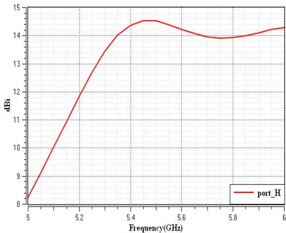
水平 (Horizontal) Gain
