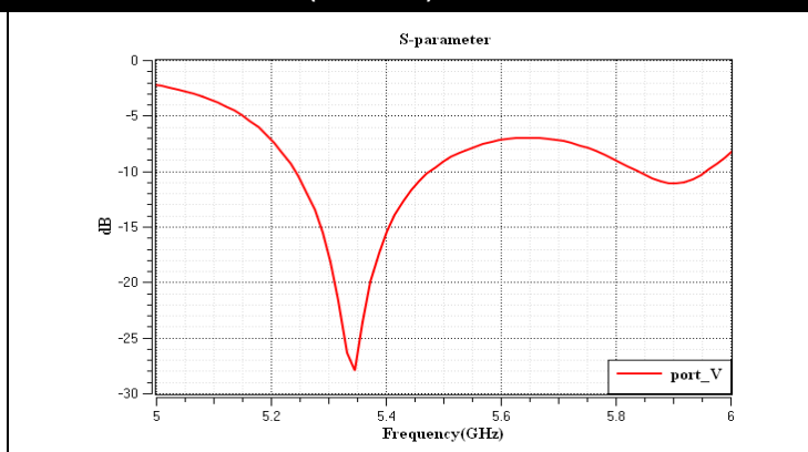
垂直 (Vertical) Return Loss
