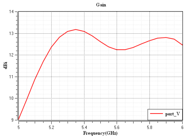
垂直 (Vertical) Gain
