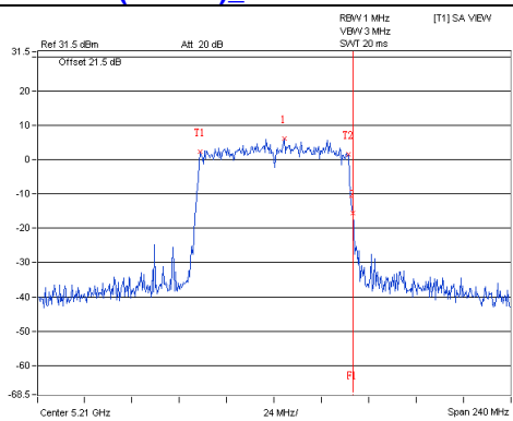
802.11ac(VHT80)_Chain2 / CH42
