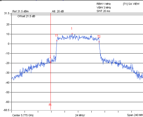
802.11ac(VHT80)_Chain1 / CH155
