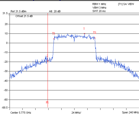
802.11ac(VHT80)_Chain2 / CH155
