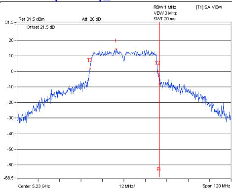
802.11ac(VHT40)_Chain2 / CH46
