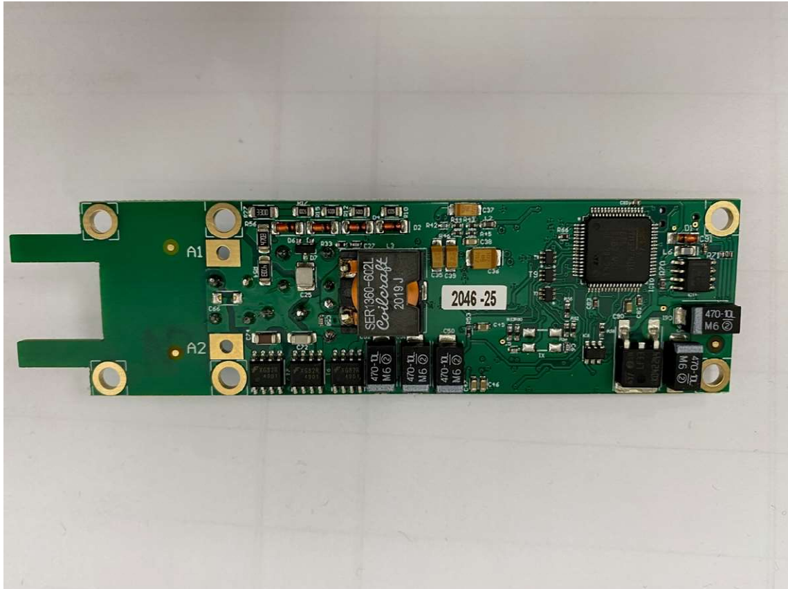
ISO_Module0.03.PCB BOTTOM
