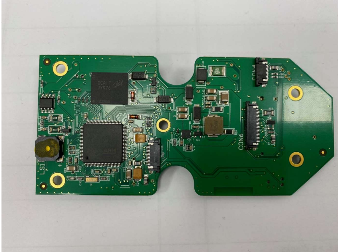
HHR5000.0.05.PCB BOTTOM
