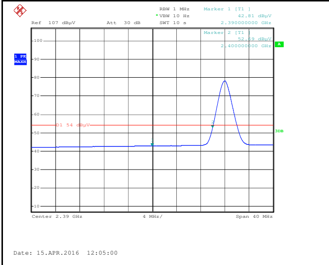
Band Edge, Left Side (Average)
