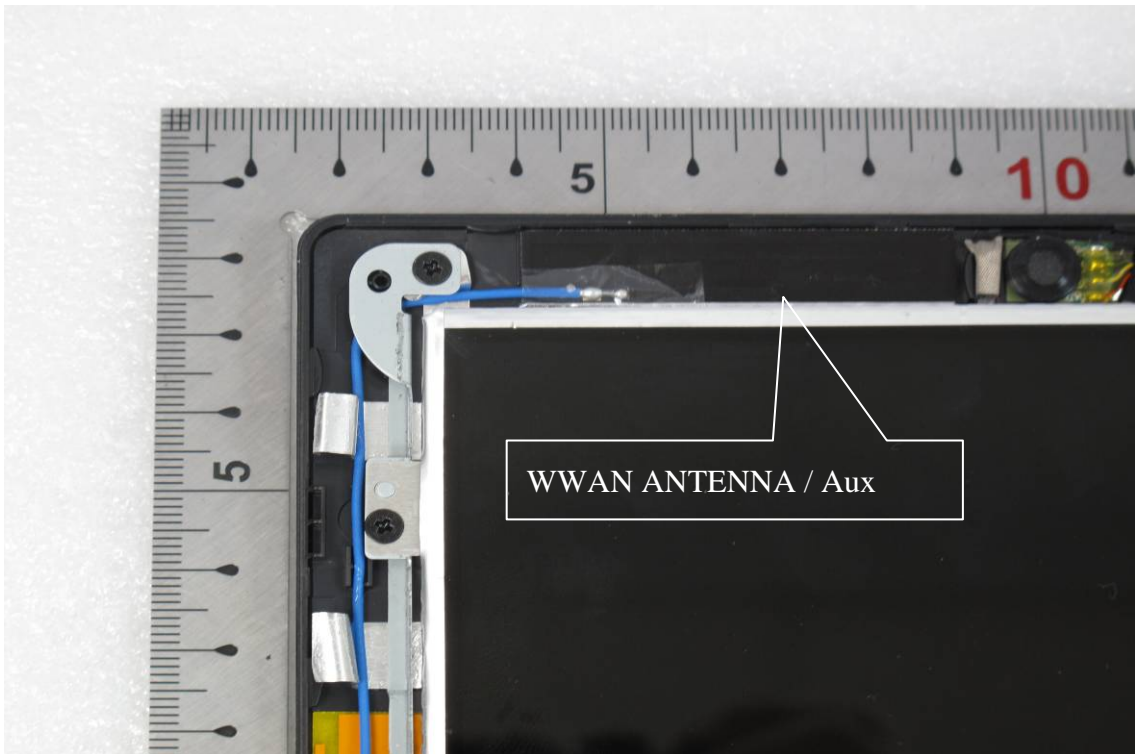
Antenna- Left
