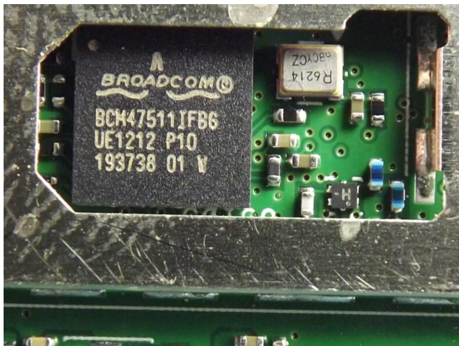
GPS Module
