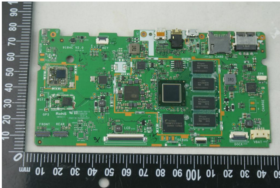
EUT Photo 8
