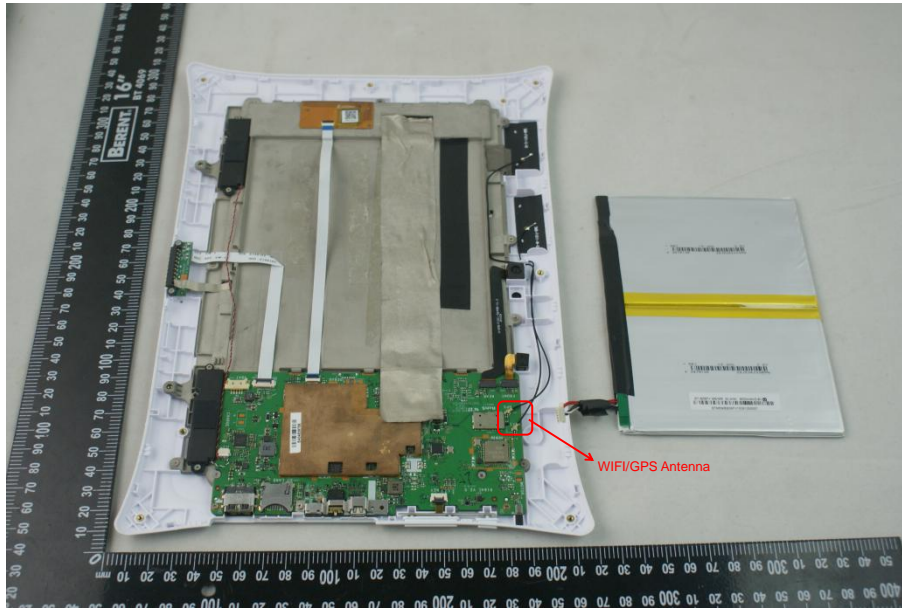
EUT Photo 3
