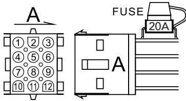
Wire Connector A:
