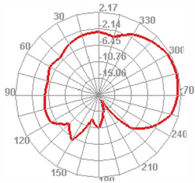
2445.000MHz E1
