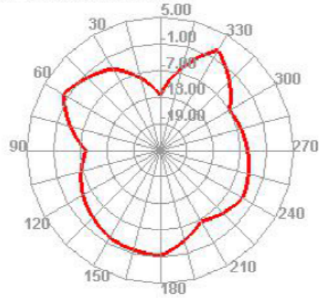
5200.000MHz H
