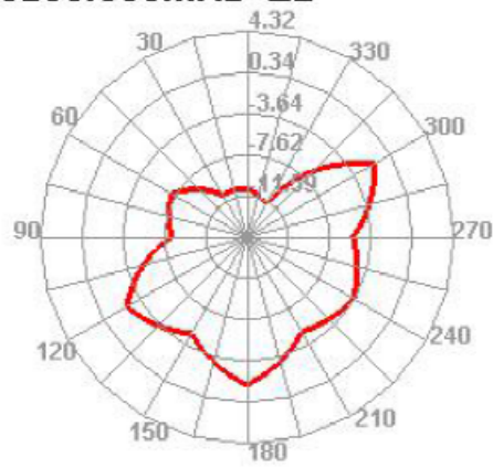
5200.000MHz E2
