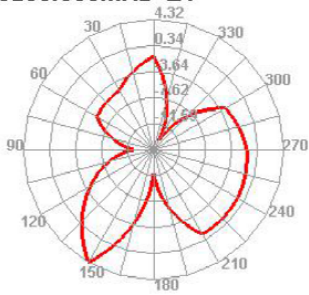
5200.000MHz E1
