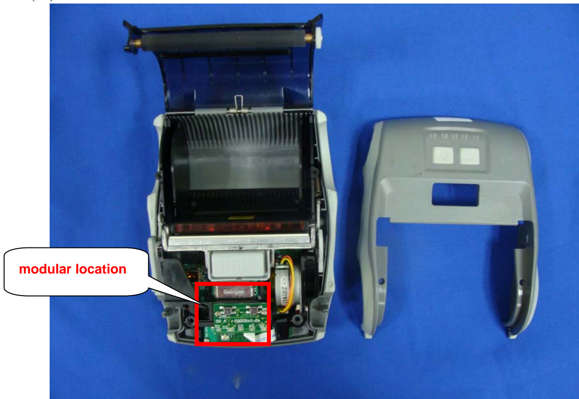
(10) EUT Photo
