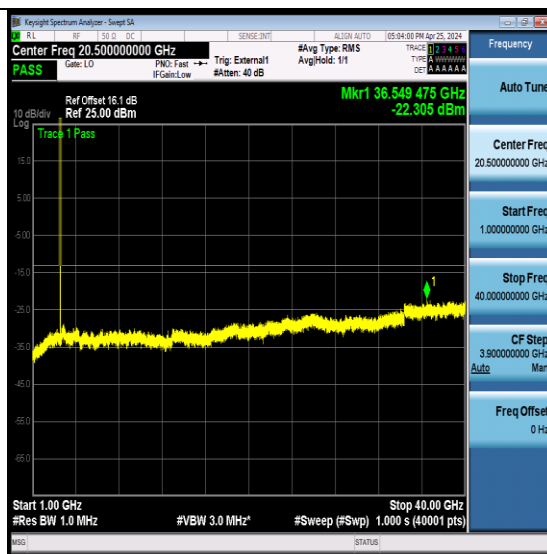
NTNV-N78-3450-3550-PC2-30-20-M-CP-QPSK- Edge_1RB_Left-Ant1-PASS
