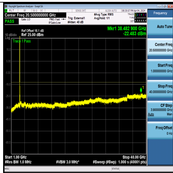
NTVN-N78-3450-3550-PC2-30-100-M-CP-QPSK- Edge_1RB_Left-Ant7-PASS
