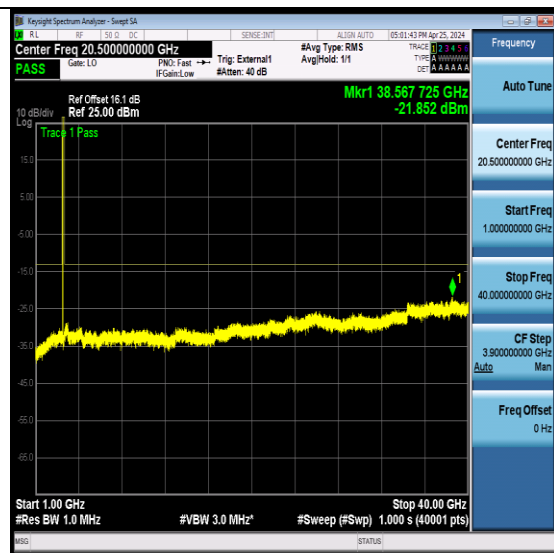
NTVN-N78-3450-3550-PC2-30-20-L-CP-QPSK- Edge_1RB_Left-Ant1-PASS
