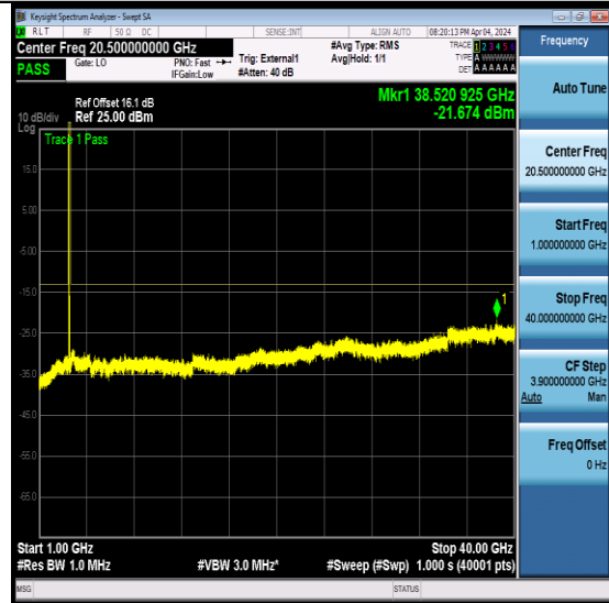
NTNV-N78-3450-3550-PC2-30-60-L-CP-QPSK- Edge_1RB_Left-Ant7-PASS
