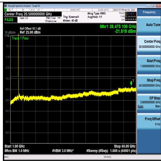
NTNV-N78-3450-3550-PC2-30-20-H-CP- QPSK-Edge_1RB_Left-Ant7-PASS
