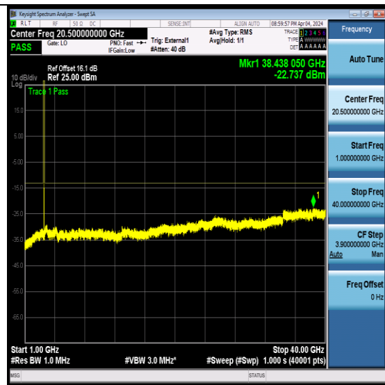
NTNV-N78-3450-3550-PC2-30-60-M-CP-QPSK- Edge_1RB_Left-Ant7-PASS
