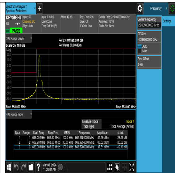
NTNV-N71-PC3-15-20-L-DFT-QPSK-Edge_1RB_Left-Ant0-PASS
