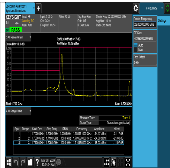
NTVN-N66-PC3-15-15-L-DFT-QPSK-Edge_1RB_Left-Ant0-PASS
