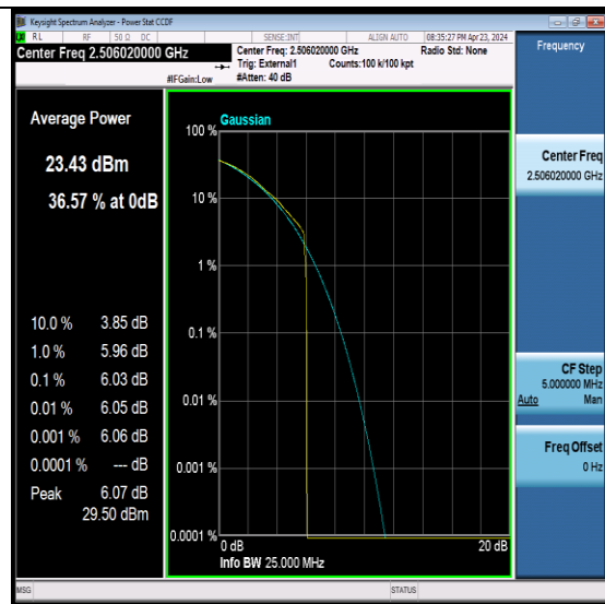
NTNV-N41-PC2-30-20-L-CP-QPSK-Edge_1RB_Left-PASS
