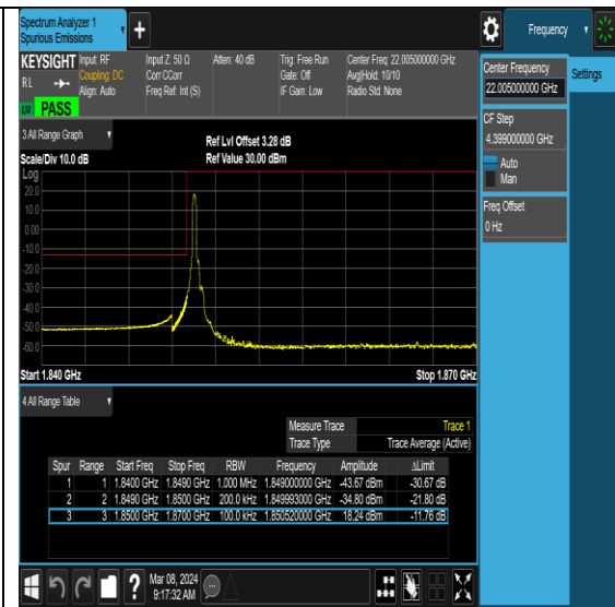
NTNV-N25-PC3-15-20-L-DFT-QPSK-Edge_1RB_Left-Ant0-PASS
