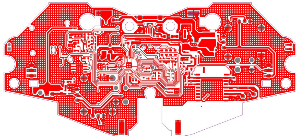
Top Layer
