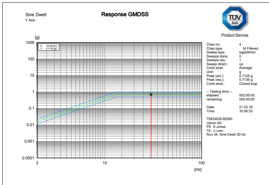
Y axis endurance run (EUT plot)
