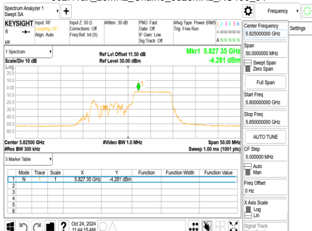
802.11ax_20MHz_Chain0_5825MHz_RU26_8
