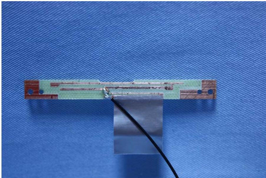
(18) EUT Photo(M/N:M760J)
