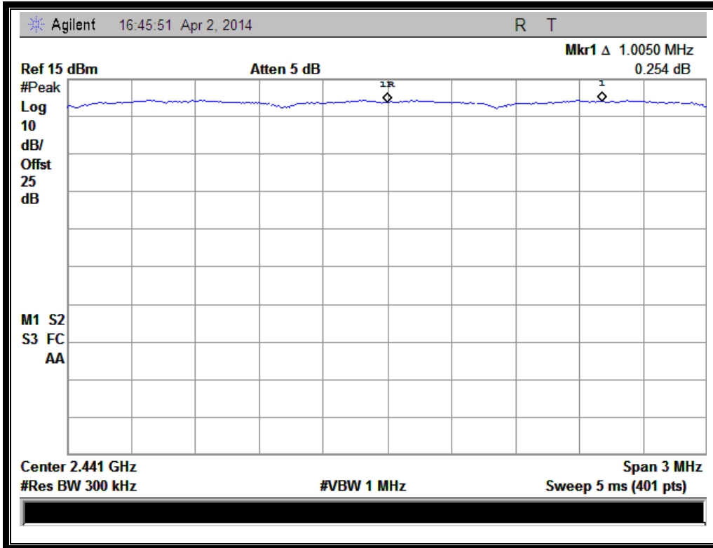
(Plot B: □/4-QPSK)
