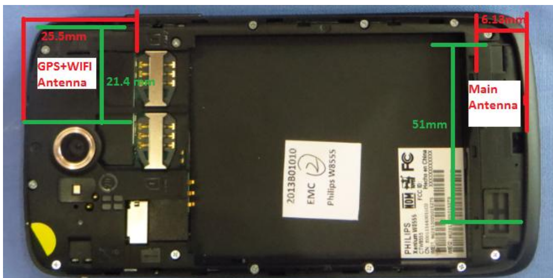
EUT
