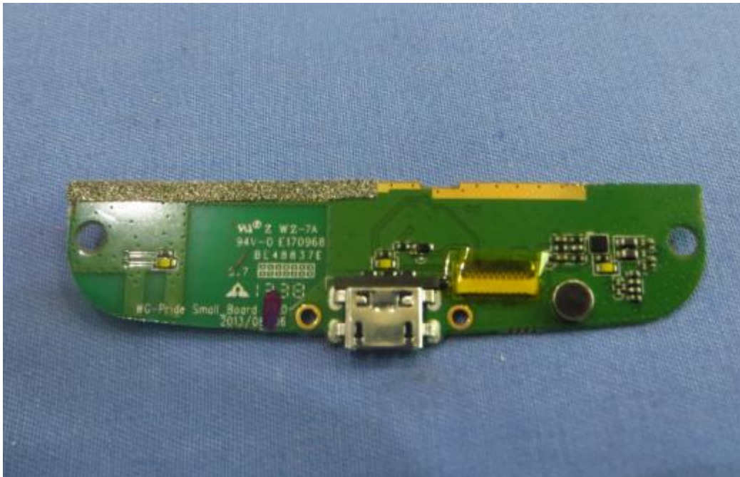
EUT
