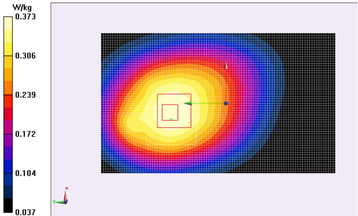
Fig.6 WCDMA 850
