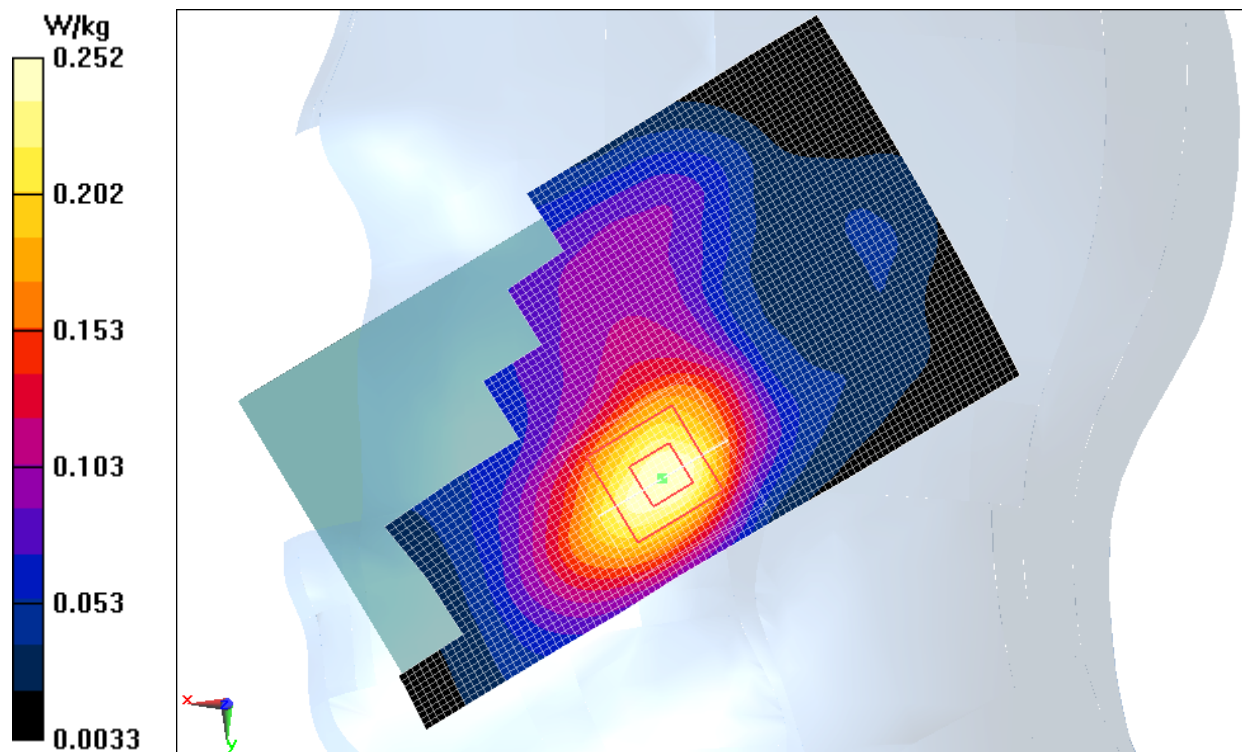
Fig.7 WCDMA1900 CH9538
