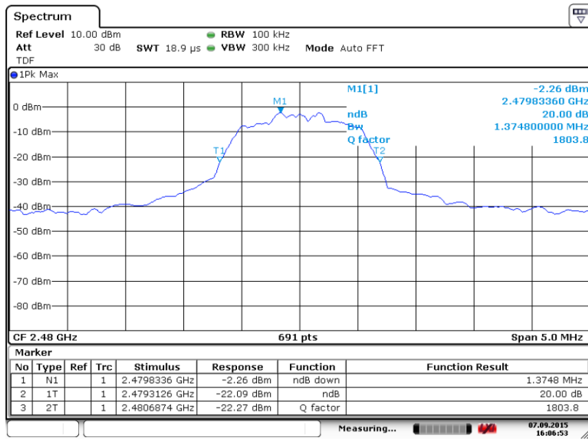
Fig. 77 Occupied 20dB Bandwidth ( \pi/4 DQPSK, Ch 78)
