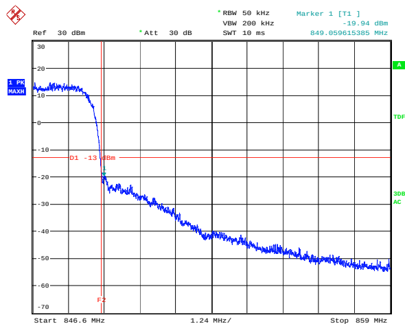
Top Band Edge (HSDPA)
