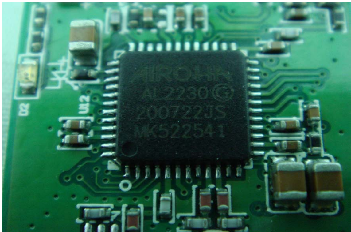
RF Module
