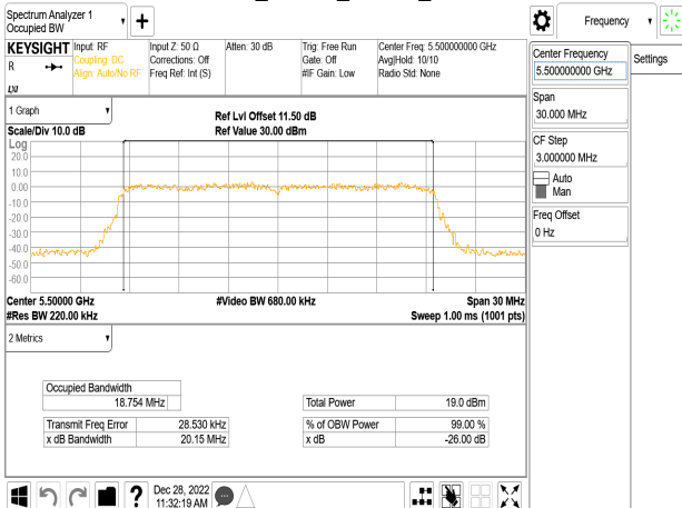
802.11ax_20MHz_Chain0_5500MHz
