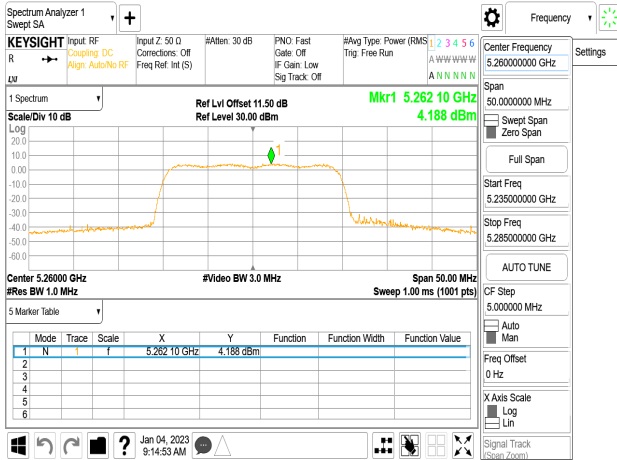
802.11ax_20MHz_Chain0_5260MHz_SU
