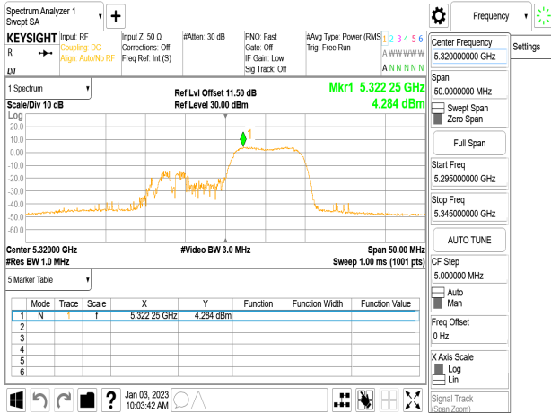
802.11ax_20MHz_Chain0_5320MHz_RU26_0
