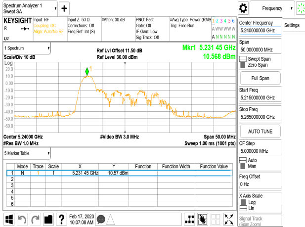
802.11ax_20MHz_Chain0_5240MHz_RU26_8
