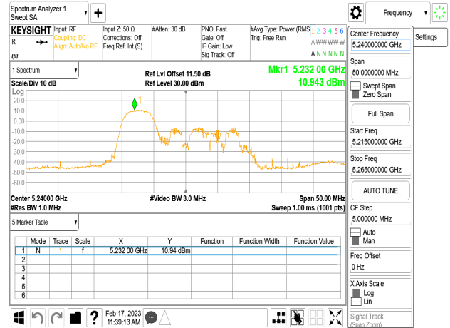
802.11ax_20MHz_Chain0_5240MHz_RU52_40
