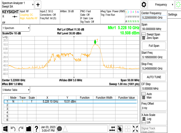
802.11ax_20MHz_Chain0_5220MHz_RU52_37
