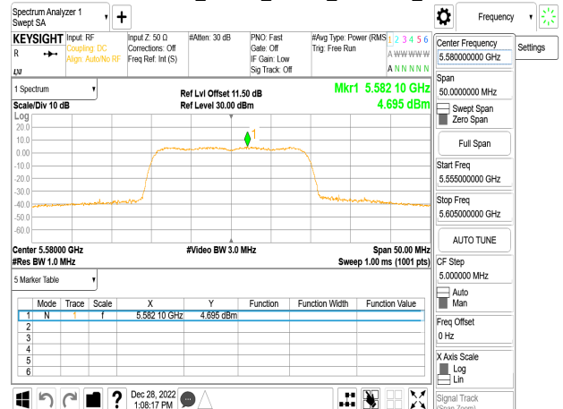
802.11ax_20MHz_Chain0_5580MHz_SU
