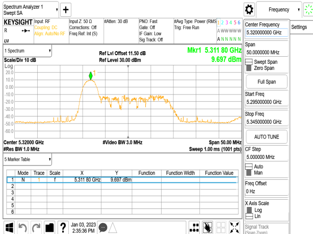
802.11ax_20MHz_Chain0_5320MHz_RU26_8
