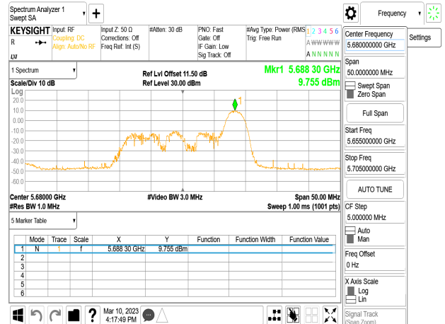
802.11ax_20MHz_Chain0_5680MHz_RU52_37
