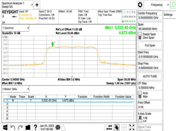
802.11ax_20MHz_Chain0_5540MHz_RU
