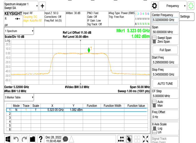
802.11ax_20MHz_Chain0_5320MHz_SU
