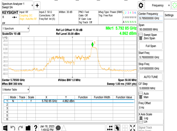
802.11ax_20MHz_Chain0_5785MHz_RU26_8
