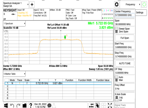
802.11ax_20MHz_Chain0_5720MHz_UNII 2C_SU
