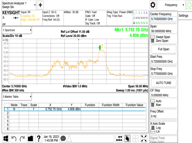
802.11ax_20MHz_Chain0_5745MHz_RU52_37
