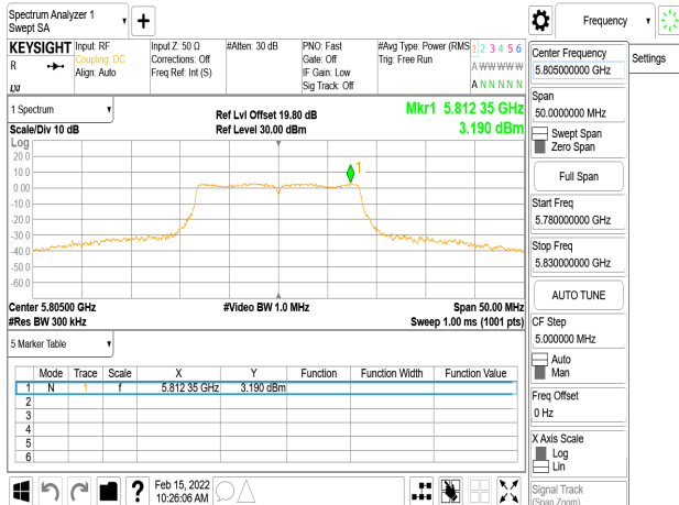
802.11a_20MHz_Chain1_5805MHz
