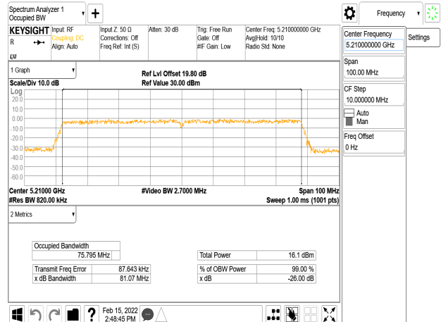
802.11ac_80MHz_Chain1_5210MHz
