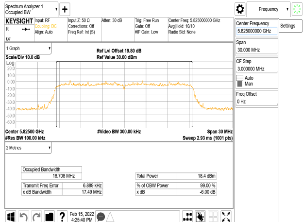
802.11ax_20MHz_Chain1_5825MHz
