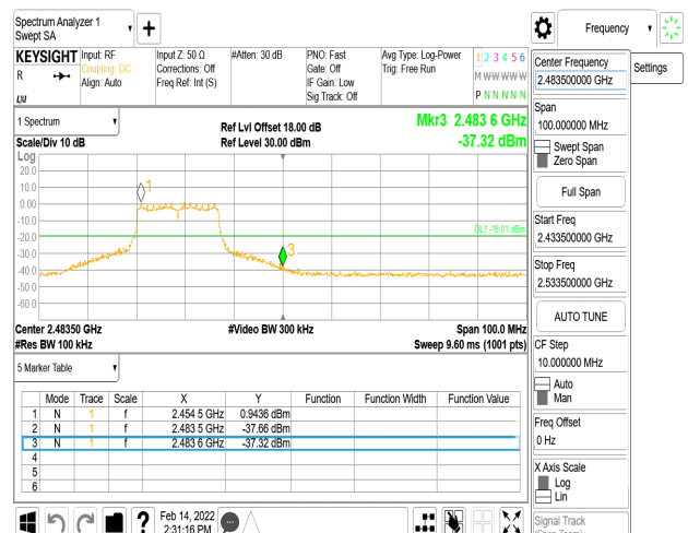
802.11g_20MHz_Chain0_2462MHz
