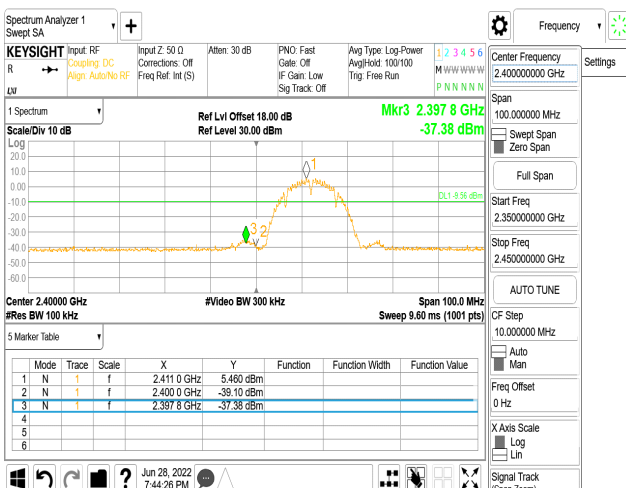
802.11b_20MHz_Chain1_2412MHz
