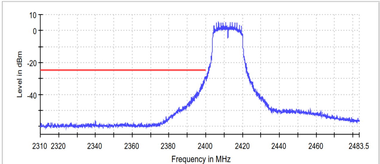
Band Edge
