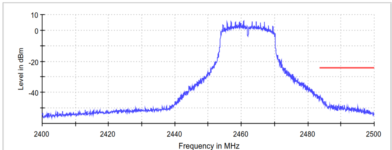
Band Edge
