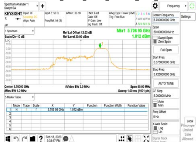
802.11ax_20MHz_Chain0_5700MHz_RU52_40
