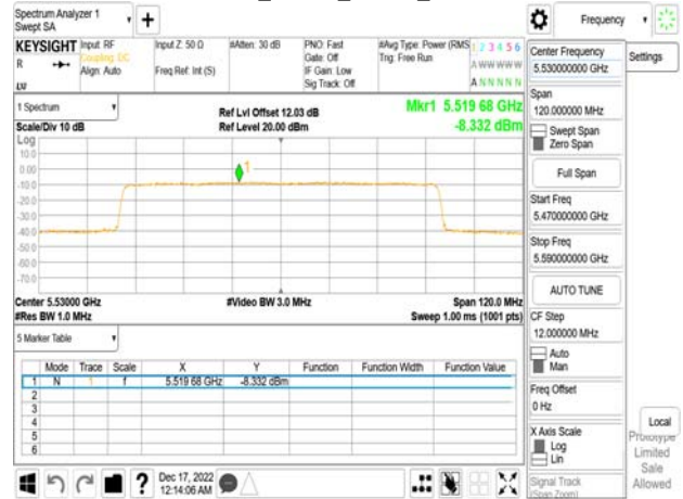
802.11ax_80MHz_Chain0_5530MHz_RU484_65
