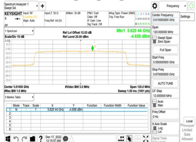
802.11ax_80MHz_Chain0_5610MHz
