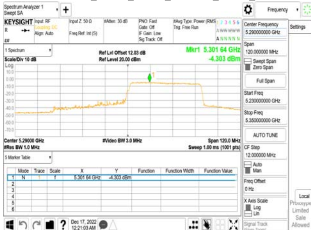
802.11ax_80MHz_Chain0_5290MHz_RU484_66
