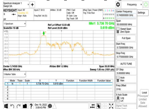
802.11ax_20MHz_Chain0_5745MHz_RU52_37
