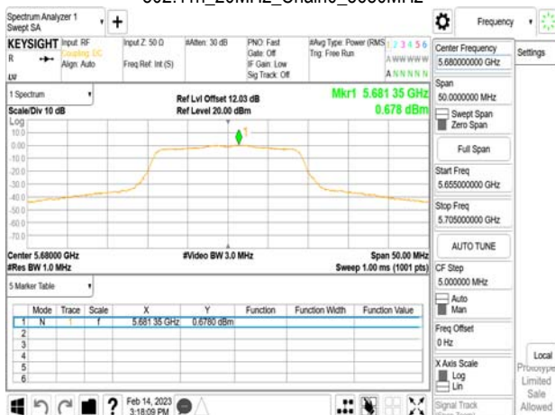
802.11n_20MHz_Chain0_5680MHz
