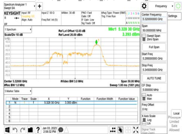
802.11ax_20MHz_Chain0_5320MHz_RU52_40
