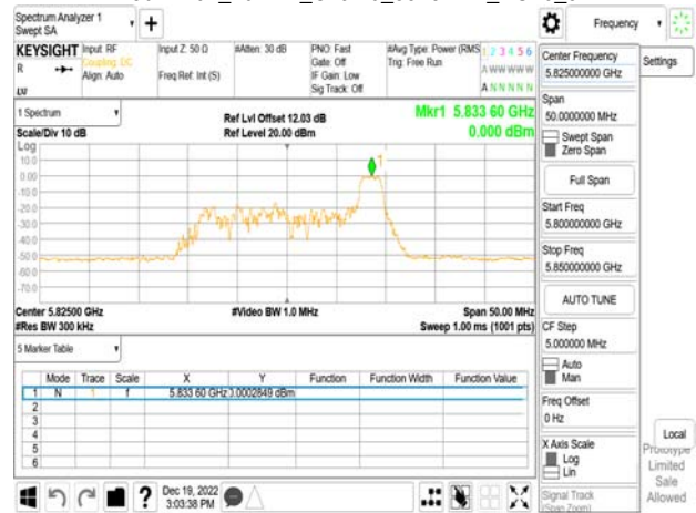
802.11ax_20MHz_Chain0_5825MHz_RU52_40
