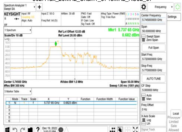
802.11ax_20MHz_Chain1_5745MHz_RU52_37
