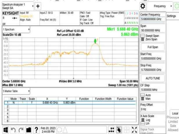
802.11ax_20MHz_Chain0_5680MHz_RU52_40
