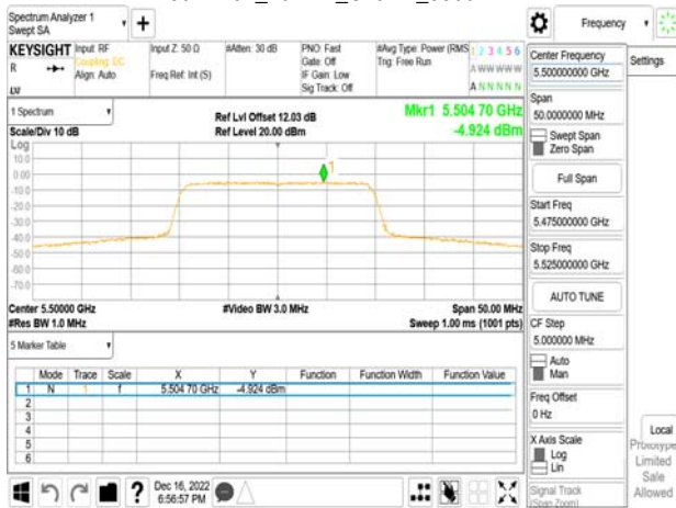
802.11ax_20MHz_Chain1_5500MHz_RU26_0
