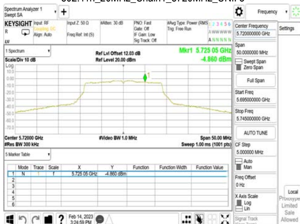
802.11n_20MHz_Chain1_5720MHz_UNII 3
