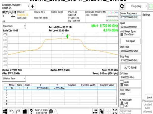
802.11a_20MHz_Chain1_5720MHz_UNII 3
