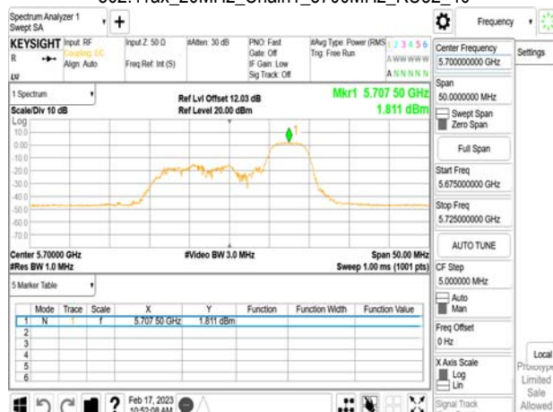
802.11ax_20MHz_Chain1_5700MHz_RU52_40
