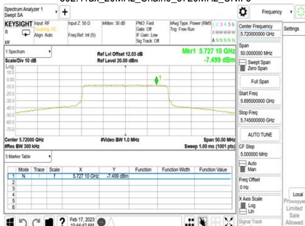
802.11ax_20MHz_Chain0_5720MHz_UNII 3
