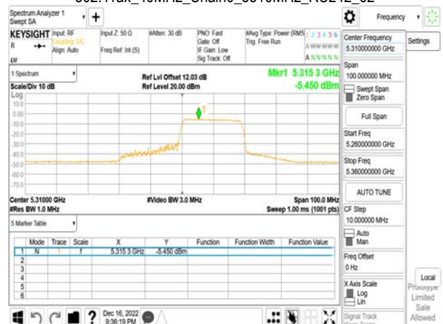
802.11ax_40MHz_Chain0_5310MHz_RU242_62
