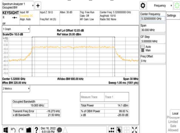
802.11ax_20MHz_Chain1_5320MHz
