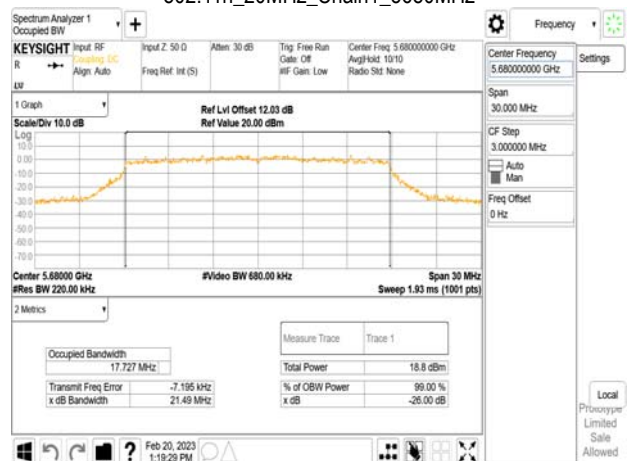
802.11n_20MHz_Chain1_5680MHz
