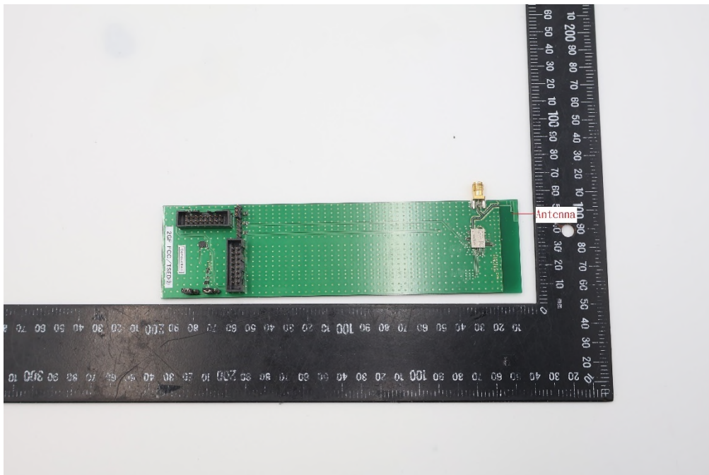
Type1LV_Antenna
