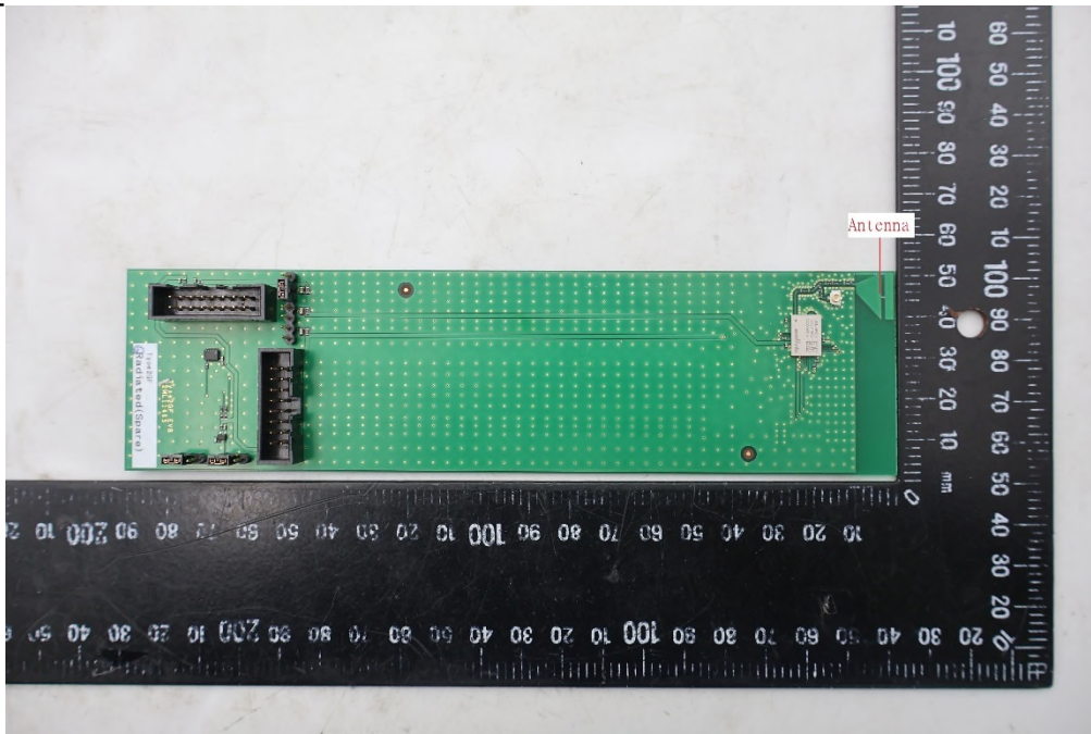
Type1LV_Antenna
