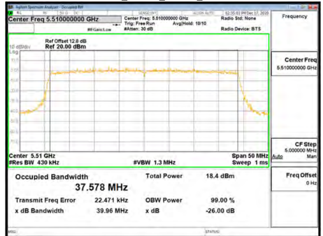
802.11ax_40MHz_Chain0_5510MHz
