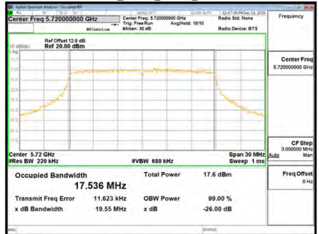
802.11n_20MHz_Chain1_5720MHz
