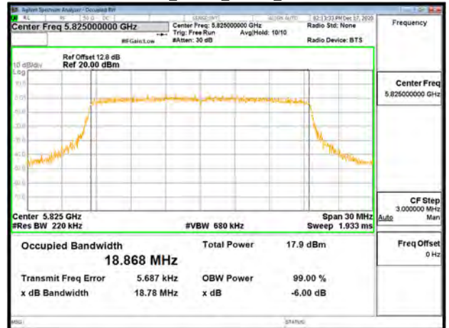
802.11ax_20MHz_Chain0_5825MHz
