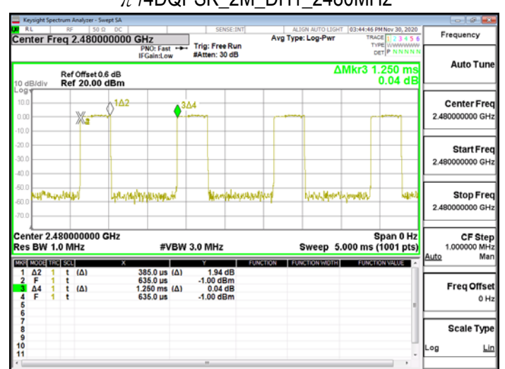
\pi /4DQPSK_2M_DH1_2480MHz
