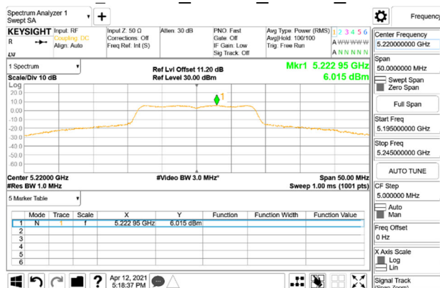
PSD_802.11a_20MHz_Chain0_5220MHz
