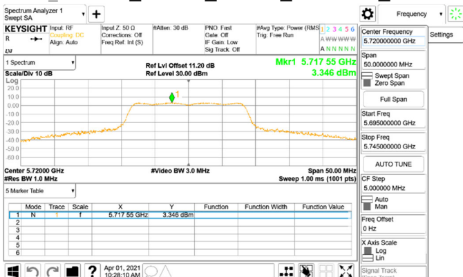
PSD_802.11a_20MHz_Chain0_5720MHz_UNII 3
