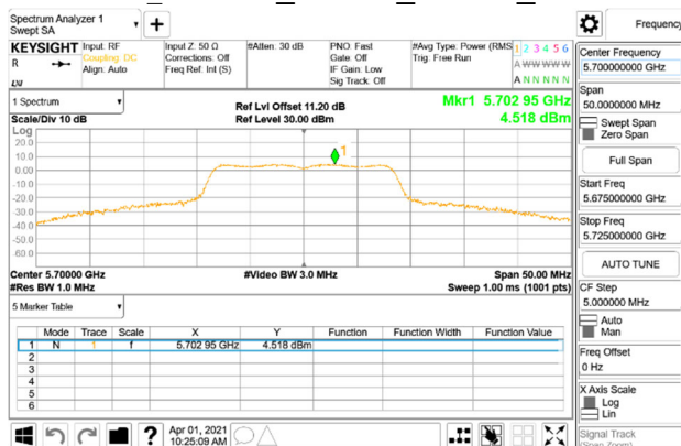
PSD_802.11a_20MHz_Chain0_5700MHz
