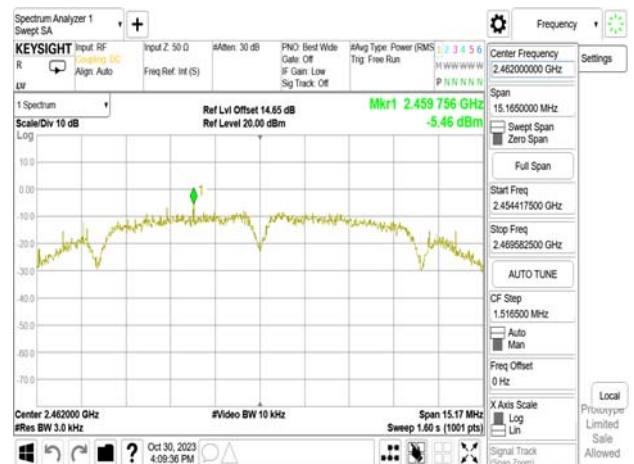
802.11b_20MHz_WLAN2_2462MHz
