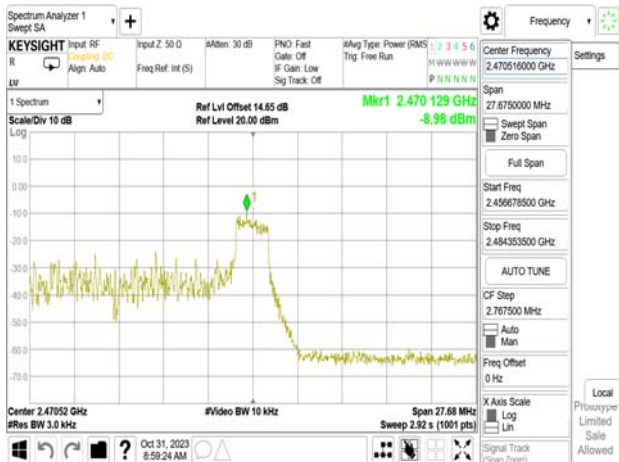
802.11ax_20MHz_WLAN1_2462MHz_RU52_40
