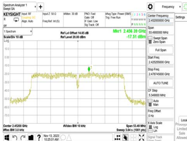
802.11n_40MHz_WLAN2_2452MHz
