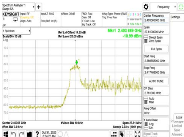
802.11ax_20MHz_WLAN1_2412MHz_RU52_37
