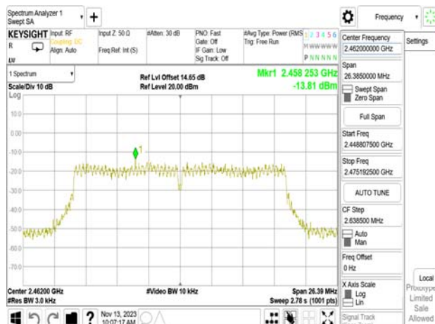
802.11n_20MHz_WLAN2_2462MHz
