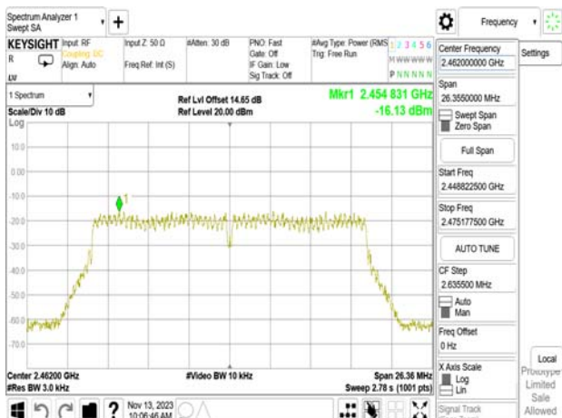
802.11n_20MHz_WLAN1_2462MHz
