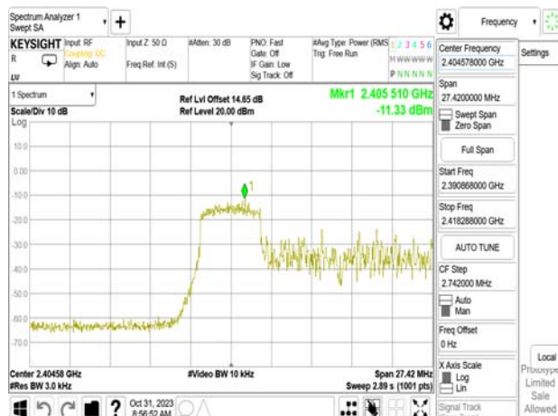
802.11ax_20MHz_WLAN2_2412MHz_RU52_37
