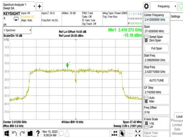
802.11ax_20MHz_WLAN2_2412MHz_RU26_0
