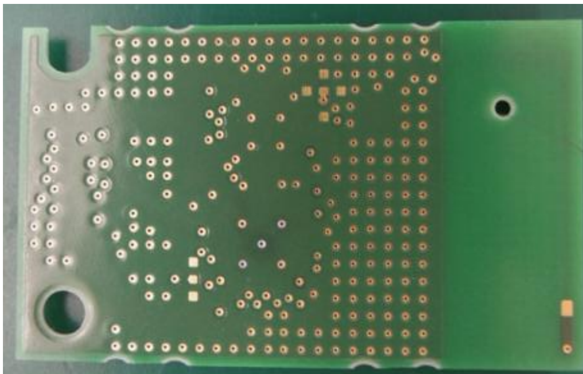
Module(Back)
