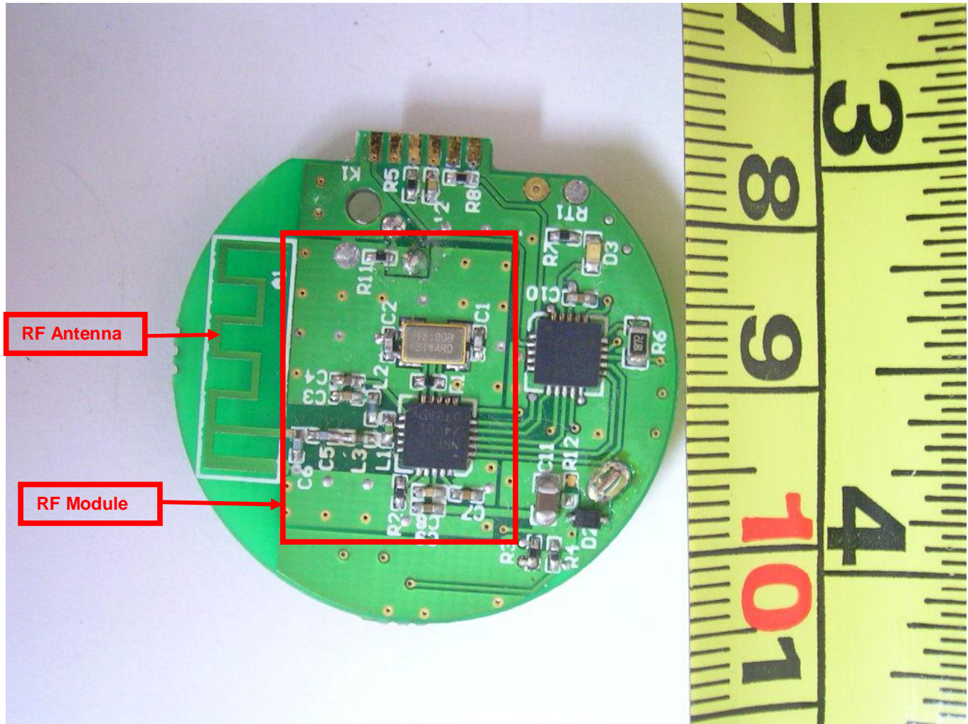
RF Module Circuit
