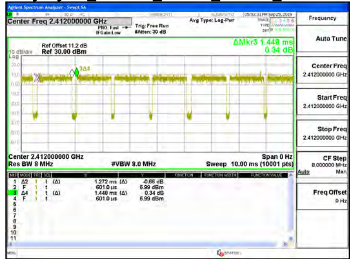
Duty Cycle 802.11n_20MHz_Chain0_2412MHz
