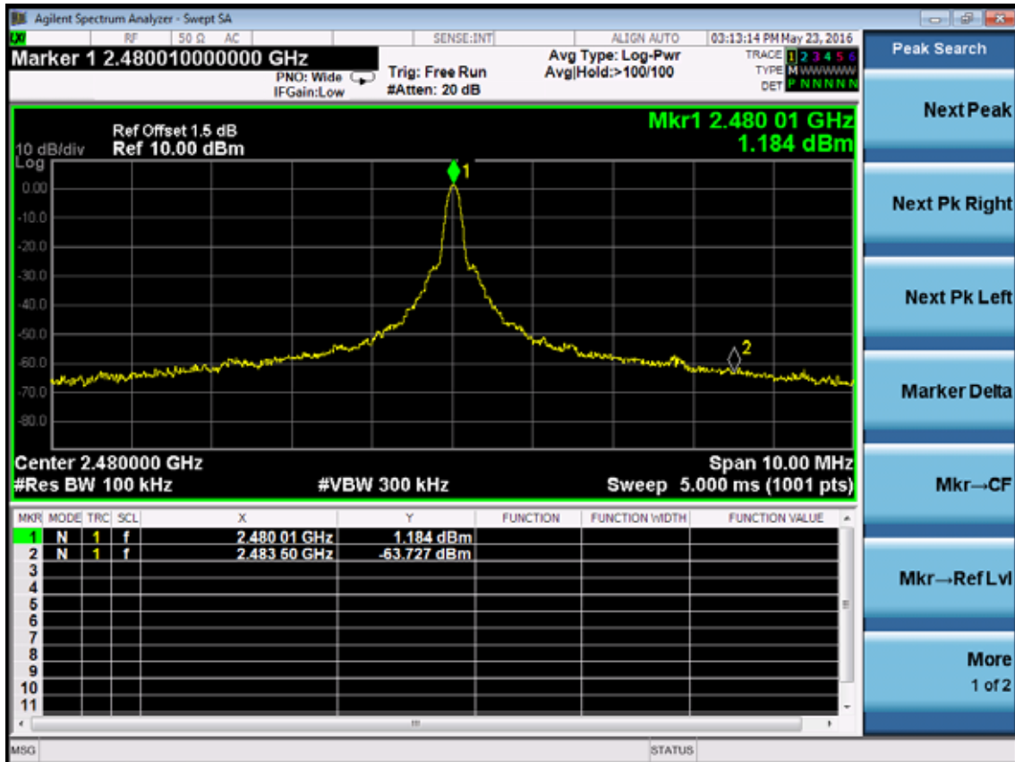
2480MHz Mark delta=64.911dB
