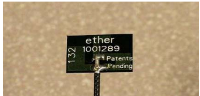
5 GHz Antenna
