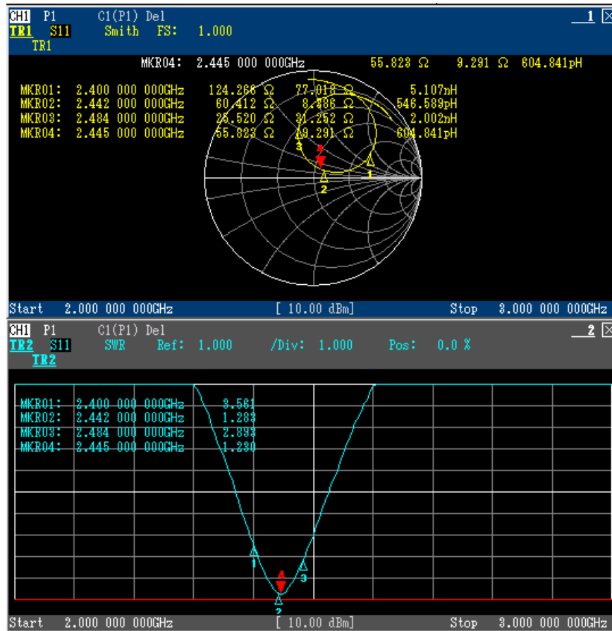
[그림 3-1] VSWR
