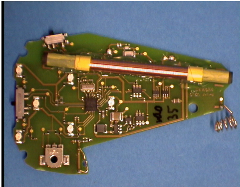
Fig. 1 PCB top
