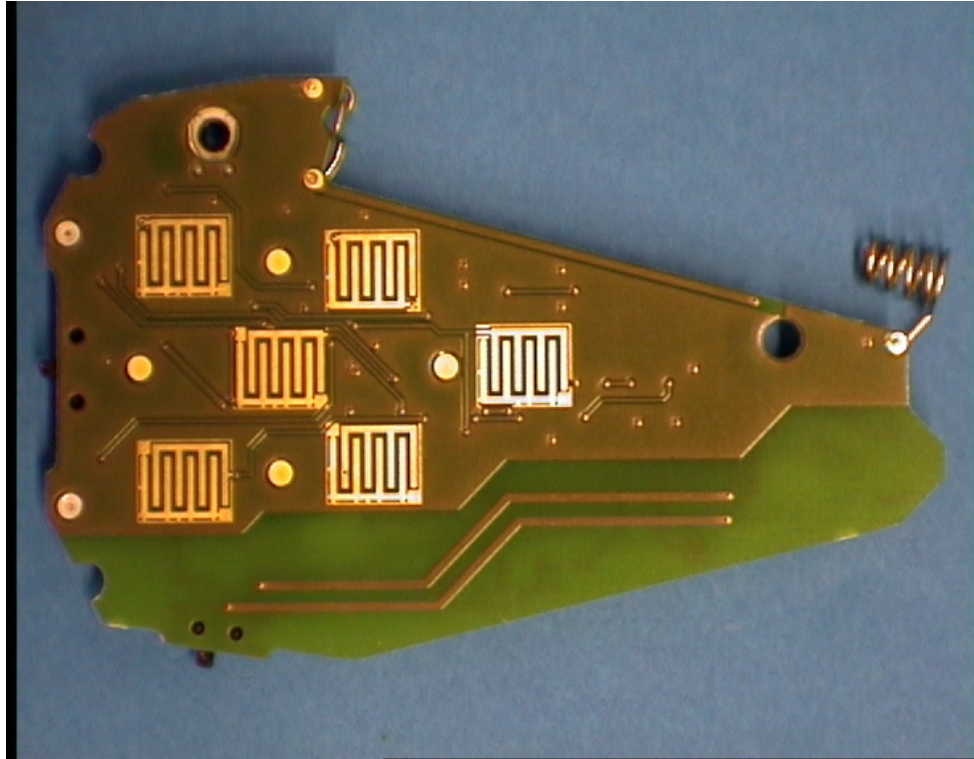
Fig. 2 PCB bottom
