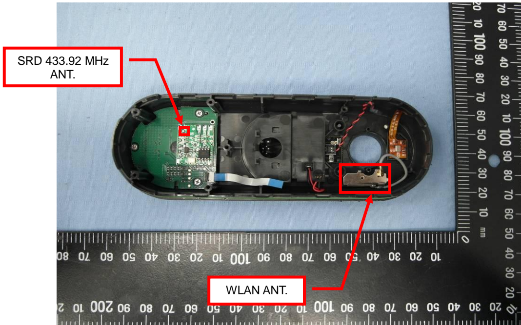
EUT Photo (20)
