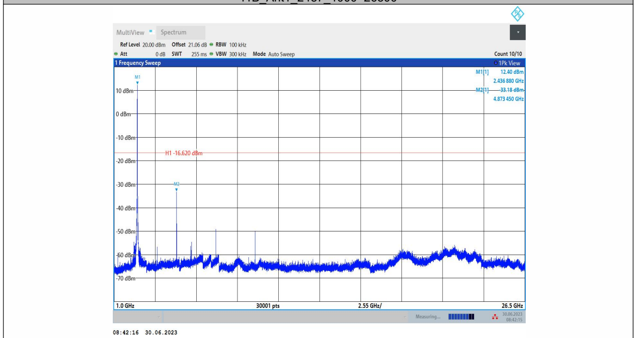
11B_Ant1_2462_0~Reference
