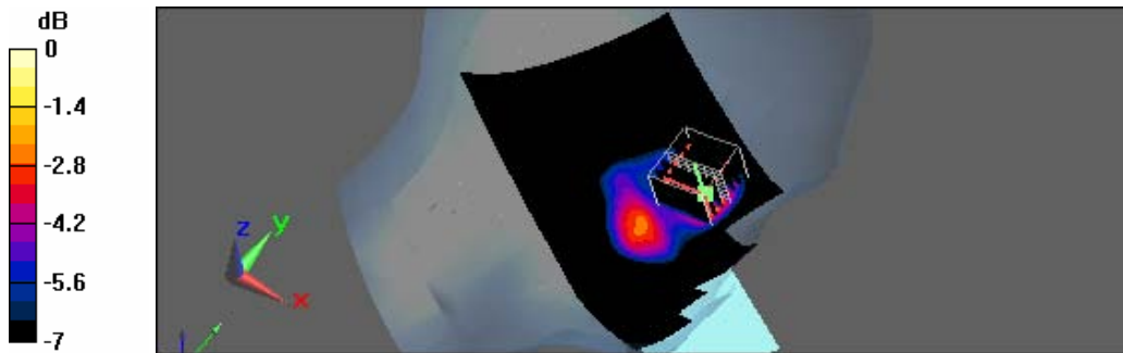
0 dB = 0.101mW/g
